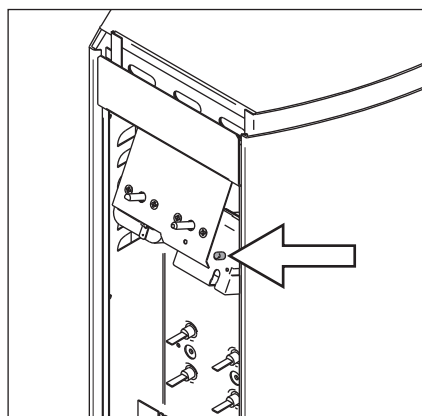
Figure 8. Reset button for overheat protector Abbildung 8. Rücksetzungsknopf des Überhitzungsschutzes
