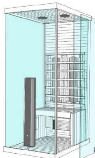
(10) Postavite šarke
